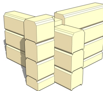
Клееный брус (соединение в «Чашку»)
